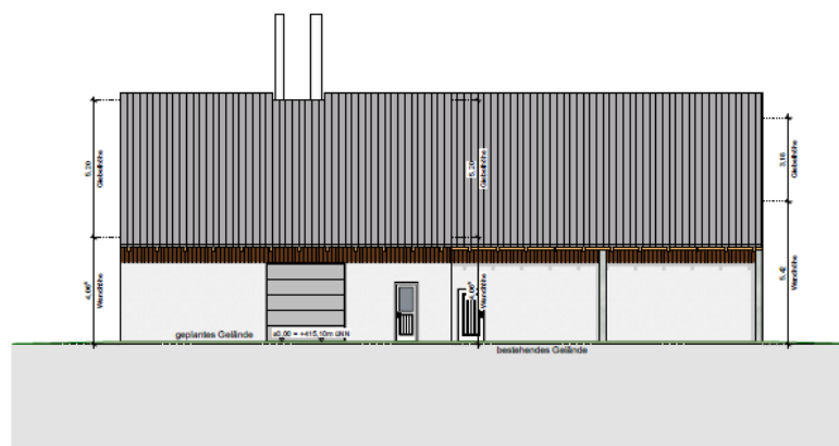
ANSICHT SÜD
